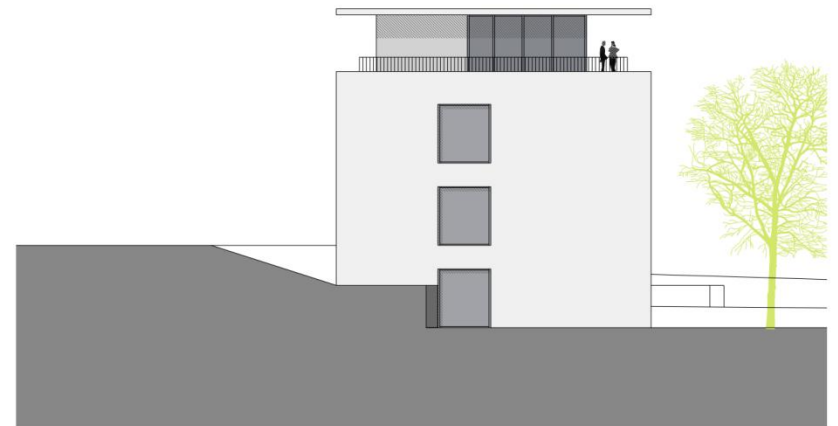
05 Ansicht West 1 : 100
