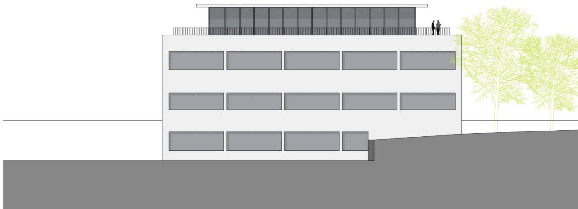
02 Ansicht Süd 1 : 100
